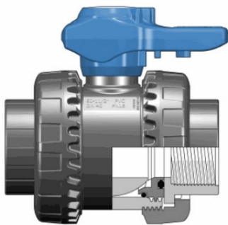
Шаровой кран ПВХ общего применения VEE; муфтовые окончания с ВР, EPDM, FIP R3/4" (DN20)
