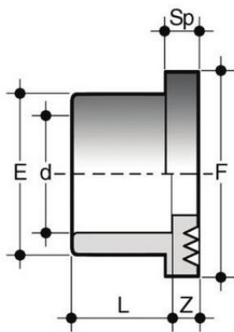
Бурт с зубчатой поверхностью ПВХ FIP d450
