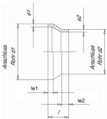
Муфта редукционная PP-H Simona (PN6) 315x250 SDR17.6 PN6
