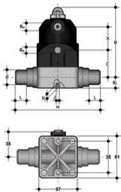
Компактный мембранный клапан СМ ПВДФ с пневмоприводом ДвД с втулочными окончаниями d20 (DN15)
