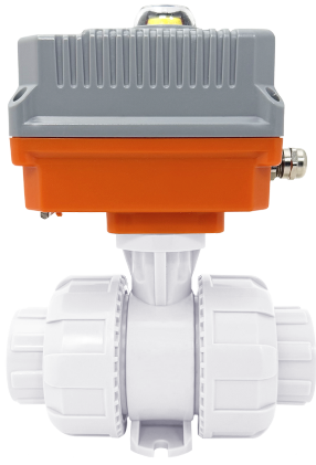
Шаровой кран IVKD ПВДФ с эл.приводом 24V DC, муфтовые окончания, EPDM, IPS d90 (DN80)
