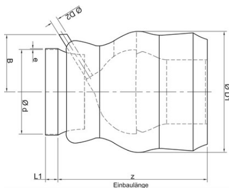
Вентилируемый кожух PPs d250
