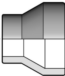
Муфта редукционная для стыковой сварки PP-H FIP 250x200 SDR11 PN6
