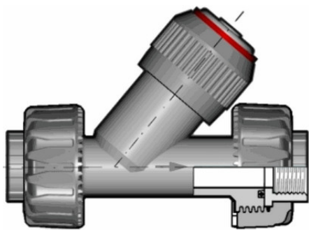
Угловой обратный клапан VRUFV ПВХ с резьбовыми окончаниями, EPDM, FIP R2" (DN50)
