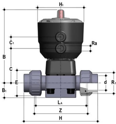
Мембранный клапан DK с пневмоприводом НО, PN10 с муфтовыми окончаниями (уплотнение EPDM/мембрана EPDM) PP-H d25 (DN20)
