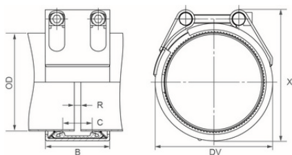
Муфта соединительная Straub-METAL-GRIP Ø180.0-609.6, NBR, W1 d406
