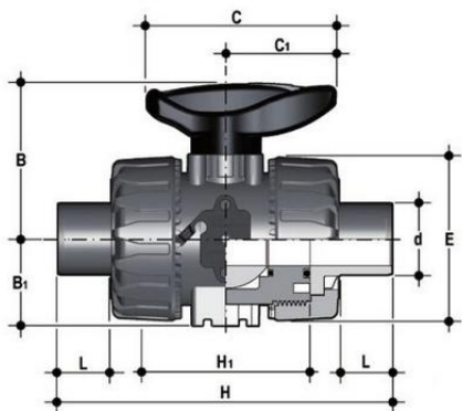
Шаровой кран VKD ПВДФ с втулочными окончаниями d50 (DN40)
