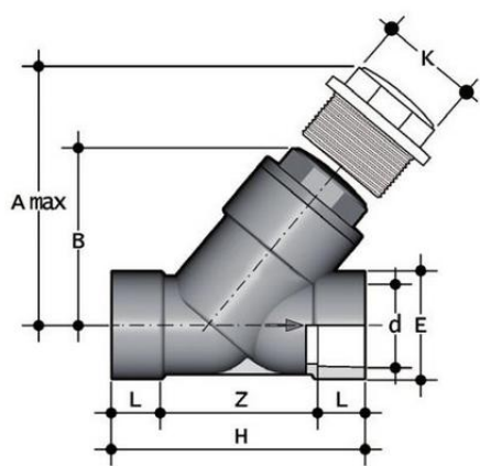
Угловой обратный клапан VRIV ПБХ с муфтовыми окончаниями, EPDM, FIP d90 (DN80)
