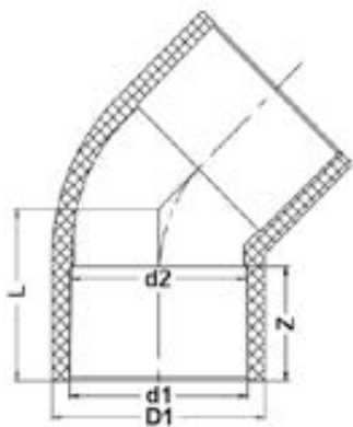
Отвод для раструбной сварки ПВДФ 45° d90 PN 16
