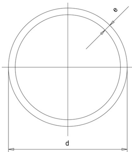
Труба ПВДФ (Simona) d125 SDR21 PN16
