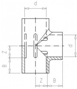
Тройник равнопроходной клеевой 90° ПВХ VDL d160
