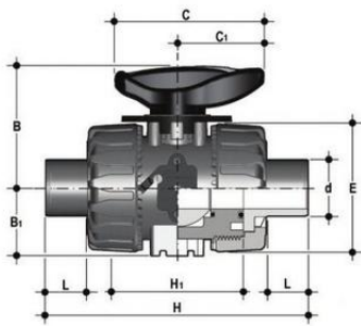
Шаровой кран для регулирования потока VKRDM с муфтовыми окончаниями (уплотнение FKM) PP-H d50 (DN40)
