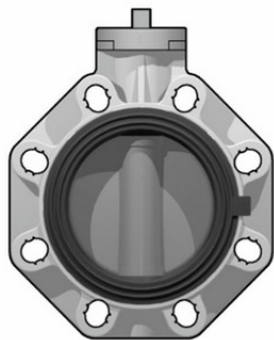
Дисковый затвор ПВХ FKOVM со свободным штоком, EPDM, FIP d355 (DN350)
