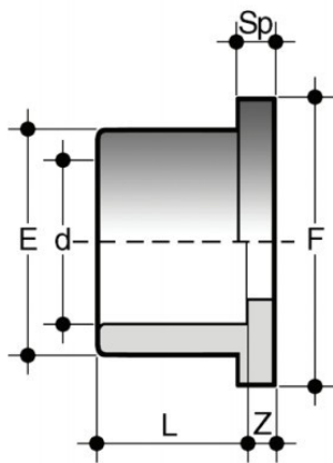
Бурт под фланец ПВХ FIP d32
