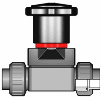
Компактный мембранный клапан CM с разборными муфтовыми окончаниями (уплотнение FKM / мембрана FKM) PP-H d20 (DN15)
