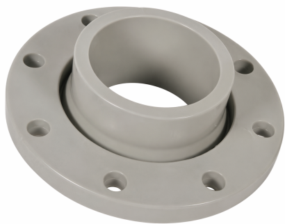
Бурт+фланец (комплект) для стыковой сварки РР-Н IPS d90 PN10
