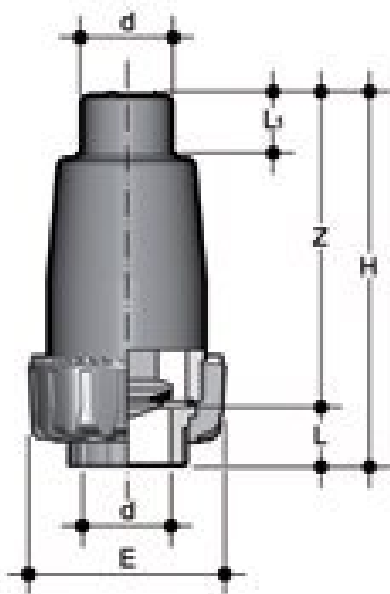
Донный клапан VZIV ПВХ с муфтовыми окончаниями, EPDM, FIP d40 (DN32)
