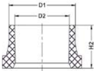
Бурт ПВДФ для стыковой сварки d25 PN 16
