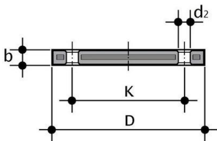
Глухой фланец PP-H FIP (PN16) d90 PN16
