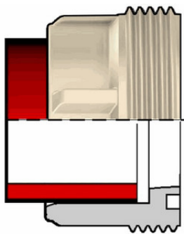
Муфтовая вставка ПВДФ d25 SDR21 PN16
