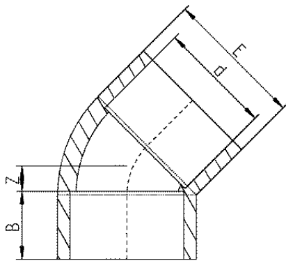
Отвод клеевой 45° ПВХ Praher Plastics d200
