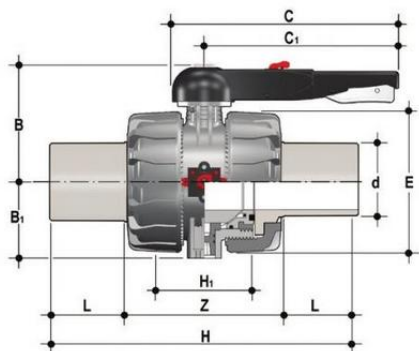
Шаровой кран VKD ПВДФ с длинными патрубками, DN65-110 d75 (DN65)
