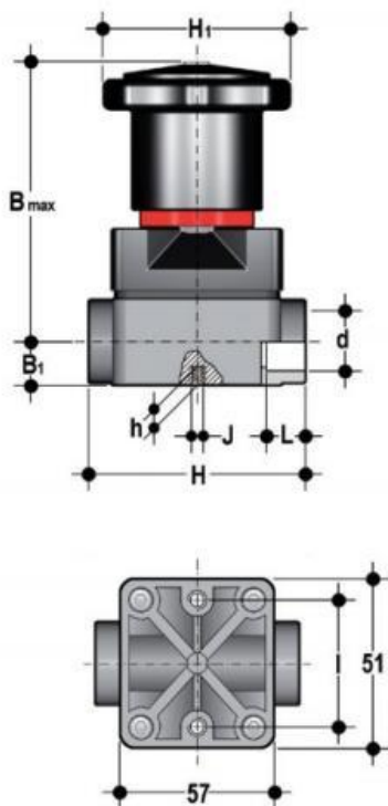
Компактный мембранный клапан ПВХ с пневмоприводом, CM, FKM, FIP d16 (DN10)
