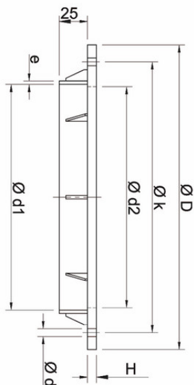
Фланцевый адаптер PPs d125
