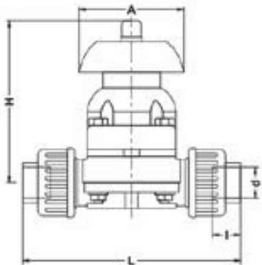
Мембранный клапан IDK ПВХ с муфтовыми окончаниями, EPDM, IPS d75 (DN65)
