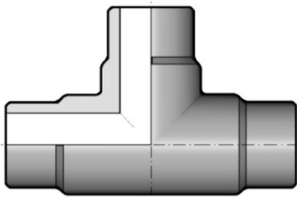
Тройник равнопроходной для стыковой сварки PP-H FIP d500 SDR11 PN6
