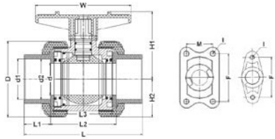
Кран шаровый ХПВХ муфтовый промышленный FKM IPS d90 (DN80)
