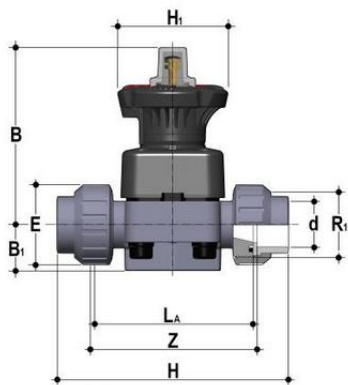
Мембранный клапан DKLUIV PBX с разборными муфтовыми окончаниями, EPDM, FIP d63 (DN50)
