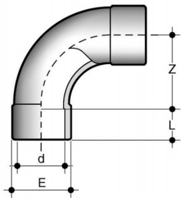
Изгиб 90° ПВХ FIP d32
