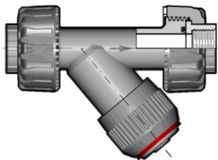
Грязевый фильтр RVUFV ПВХ с резьбовыми окончаниями, EPDM, FIP R3/8" (DN10)
