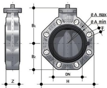
Дисковый затвор FK ПВДФ со свободным штоком d160 (DN150)
