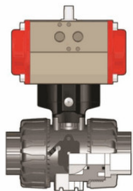
Шаровой кран VKD ПБХ с пневмоприводом ДвД с резьбовыми окончаниями, FKM, FIP R1/2" (DN15)
