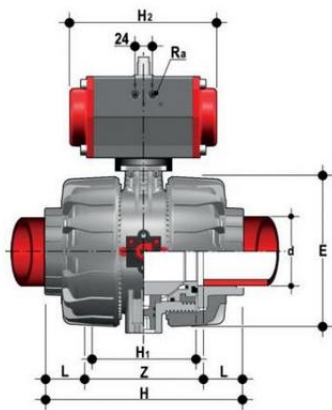
Шаровой кран VKD с пневмоприводом H3 с муфтовыми окончаниями, DN65-100 (уплотнение FKM) PP-H d90 (DN80)
