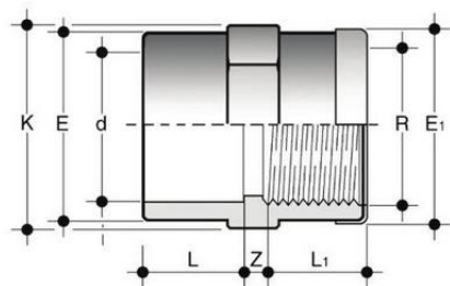
Переходная муфта с усиливающим кольцом ХПВХ 20x1/2" PN16
