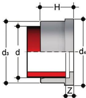
Муфтовое окончание для раструбной сварки PP-H FIP PN10
