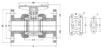
Кран шаровой промышленного применения, фланцевые окончания, FKM, IPS d63
