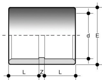
Соединительная муфта ХПВХ d25 PN16
