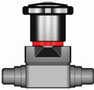
Компактный мембранный клапан CM с втулочными окончаниями (уплотнение EPDM / мембрана EPDM) PP-H d20 (DN15)
