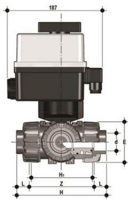
3-х ходовой шаровой кран ТКД ПБХ с эл.приводом 24V AC/DC, муфтовые окончания, Т-шар, FKM, FIP d40 (DN32)
