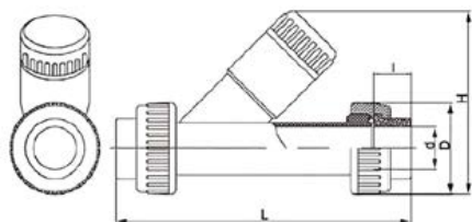
Фильтр сетчатый (грязевой) PP-H IPS d40 (DN32)
