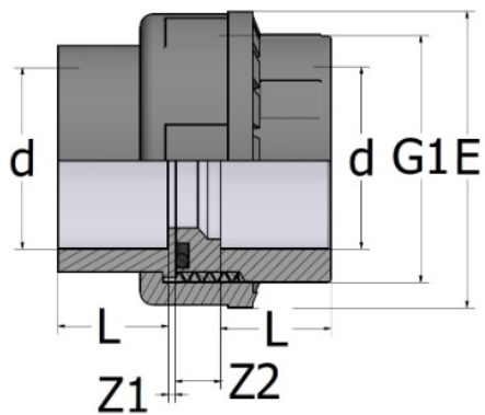
Муфта разборная ПВХ клеевая Comer d90
