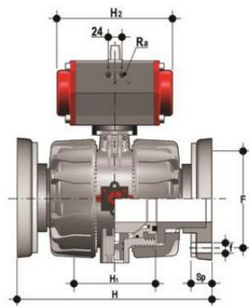
Шаровой кран VKD ПВХ с пневмоприводом ДвД с фланцевыми окончаниями, EPDM, FIP d75 (DN65)
