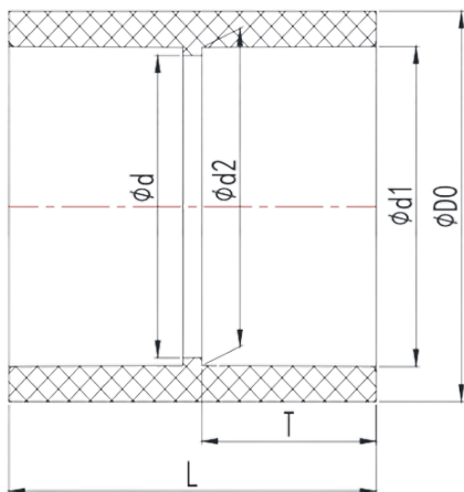
Муфта соединительная ПВХ IPS d90
