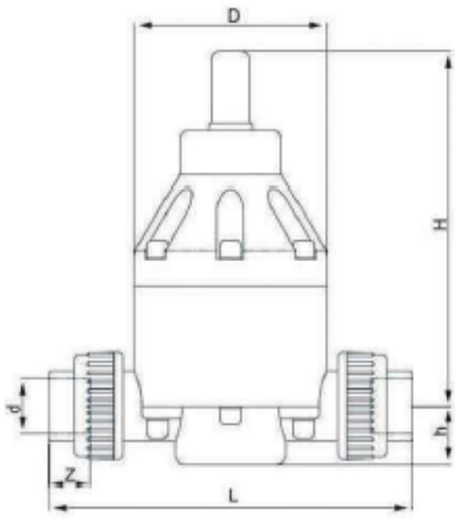
Клапан поддержания давления ПВХ с муфтовыми окончаниями, IPS d63 (DN50)
