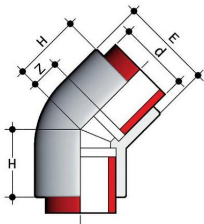
Отвод ПВДФ 45° d20 SDR21 PN16
