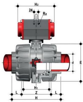
Шаровой кран VKD с пневмоприводом ДвД с муфтовыми окончаниями, DN65-100 (уплотнение FKM) PP-H d75 (DN65)
